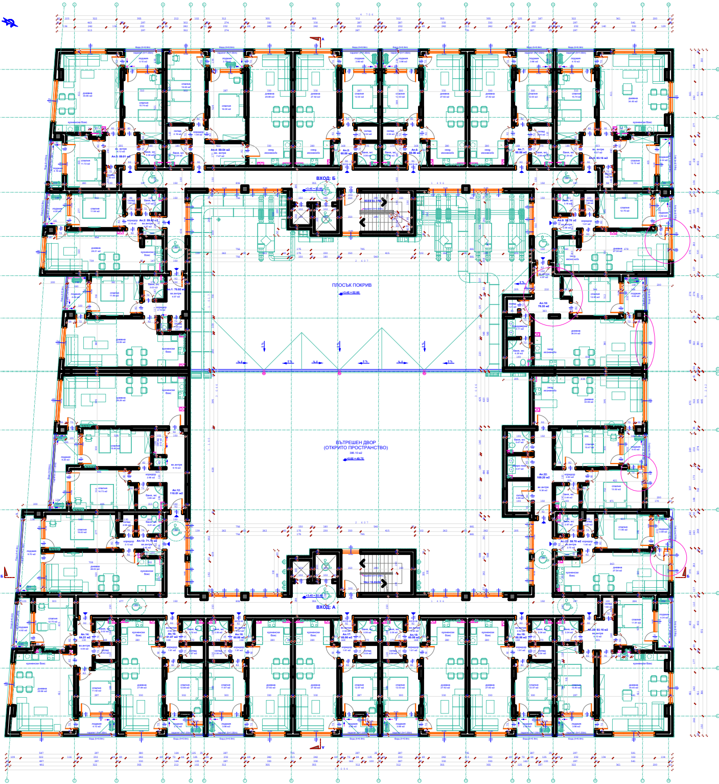
РАЗПРЕДЕЛЕНИЕ НА ЕТАЖ 2 (КОТА +3.45) Площ: 11 620,97 кв.м
