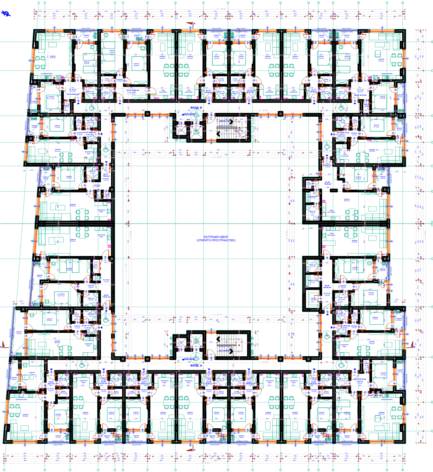
РАЗПРЕДЕЛЕНИЕ НА ЕТАЖ 3 (КОТА +6.30) Проект 1:000/87 м 2
