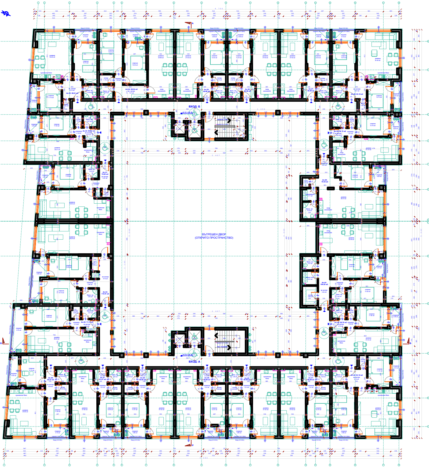
РАЗПРЕДЕЛЕНИЕ НА ЕТАЖ 4 (КОТА +9.15) Проект 1:000:87.02
