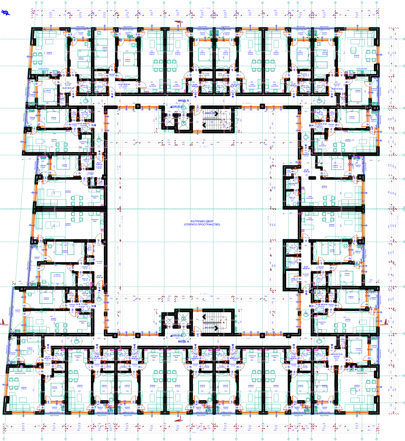
РАЗПРЕДЕЛЕНИЕ НА ЕТАЖ 5 (КОТА +12.00) Фиг. 1 (00/07/20)
