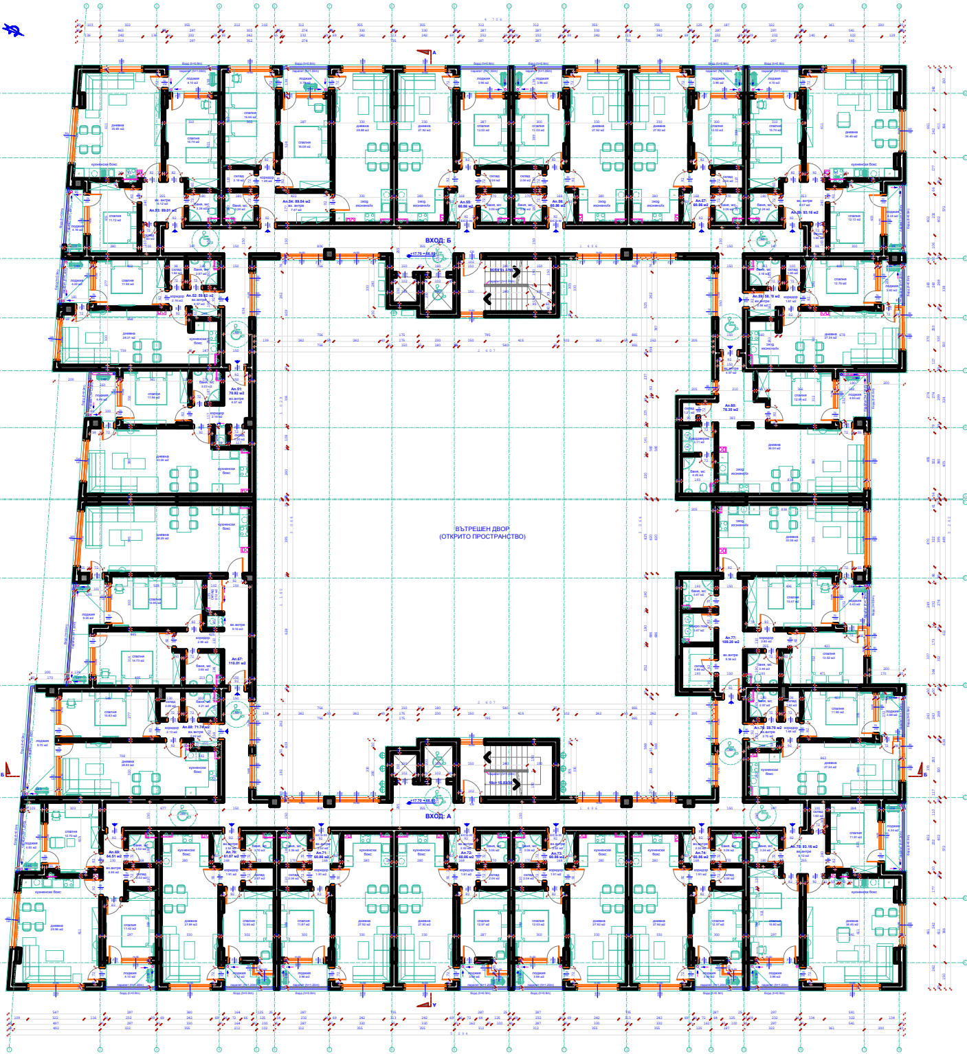
РАЗПРЕДЕЛЕНИЕ НА ЕТАЖ 7 (КОТА +17.70) Формат: А3 (841x1189)
