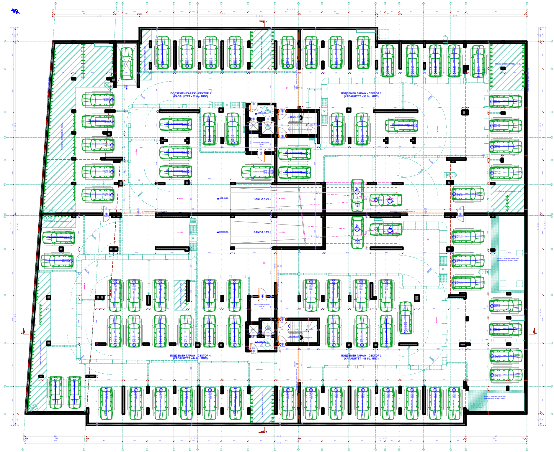
РАЗПРЕДЕЛЕНИЕ НА СУТЕРЕН (КОТА: -6.15) Треша 2.102.01.01
